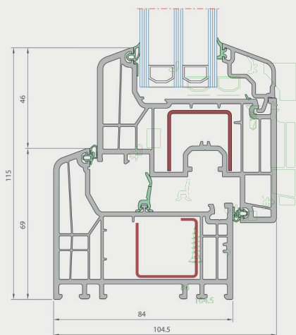
Przekrój pionowy
